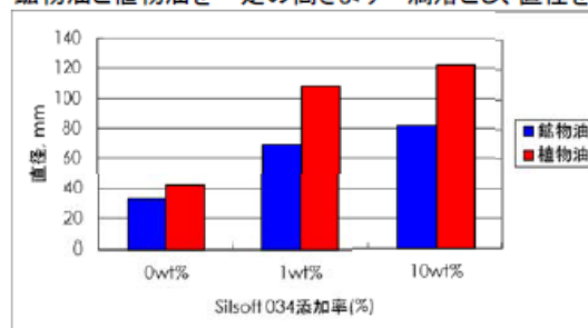
拡がり性の確認: 鉱物油と植物油を一定の高さより一滴落とし、直径を確認。
