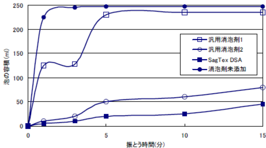
図1. 振とう試験機による消泡試験(発泡液:0.5%ドデシルベンゼンスルホン酸)
